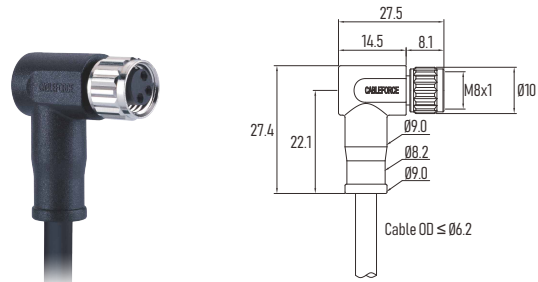
90° Right Angled 弯头
